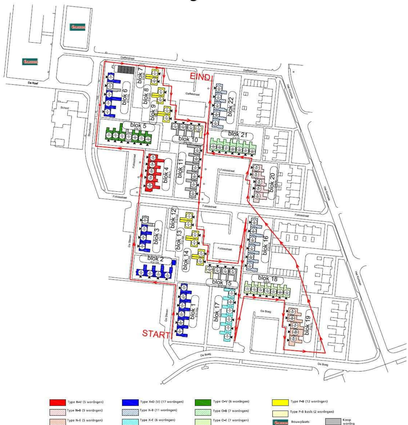
Figuur 7 Bouwroute
