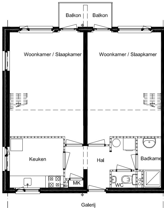
Begane Grond
